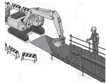
土止め先行工法
